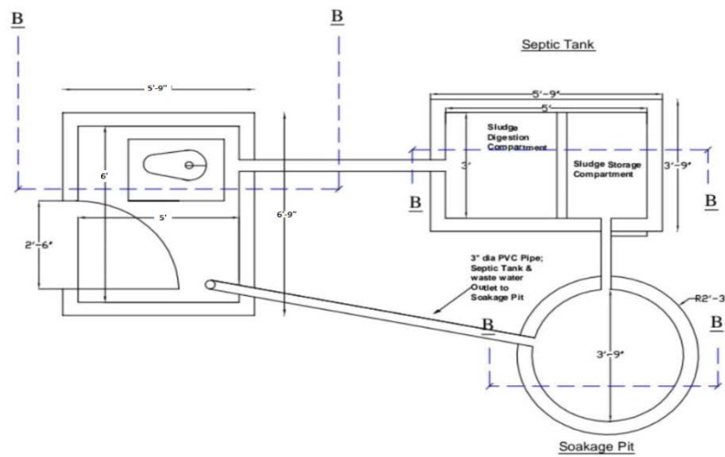
Plan Pour Flush Latrine 6'x5'
