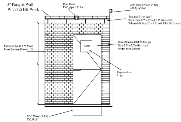
Front Elevation Pour Flush Latrine
